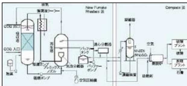
FRC法 脱硫システムフローシート
