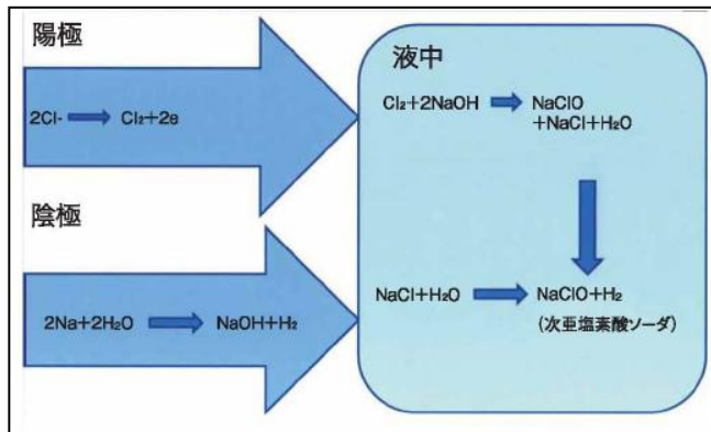
電解装置の原理(1)
