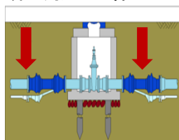
弁室周辺の配管
